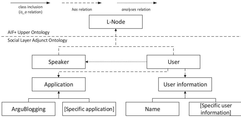
Fig. 3. AIFdb social layer AO.
