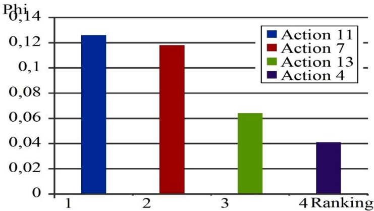
Fig. 2: Classement complet Promethee II sous contraintes
