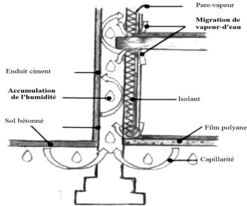
Fig. 1: Ensemble de travaux pouvant causer l'accumulation de l'humidité, adapter de [22]
