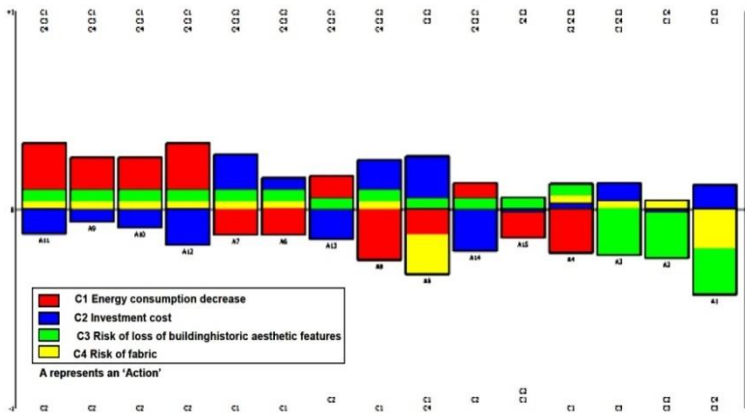
Fig. 3: Détails du flux net Phi pour toutes les actions
